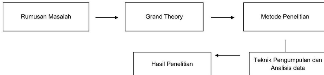
Gambar 3.1 Desain Penelitian
