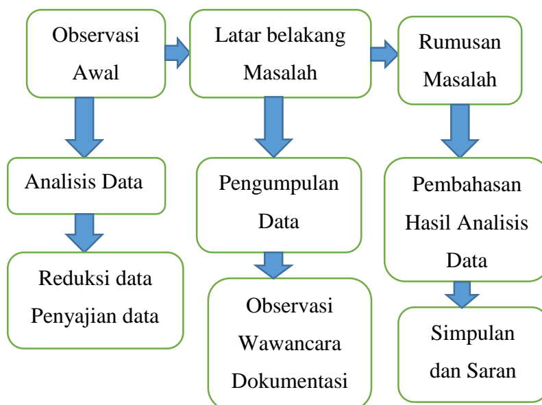
Gambar 3. 1 Desain Penelitian
