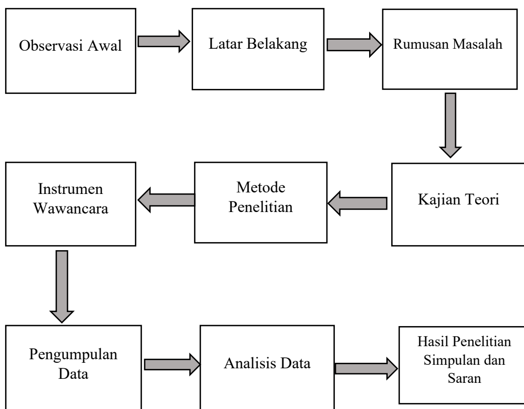
Gambar 3. 1 Desain Penelitian
