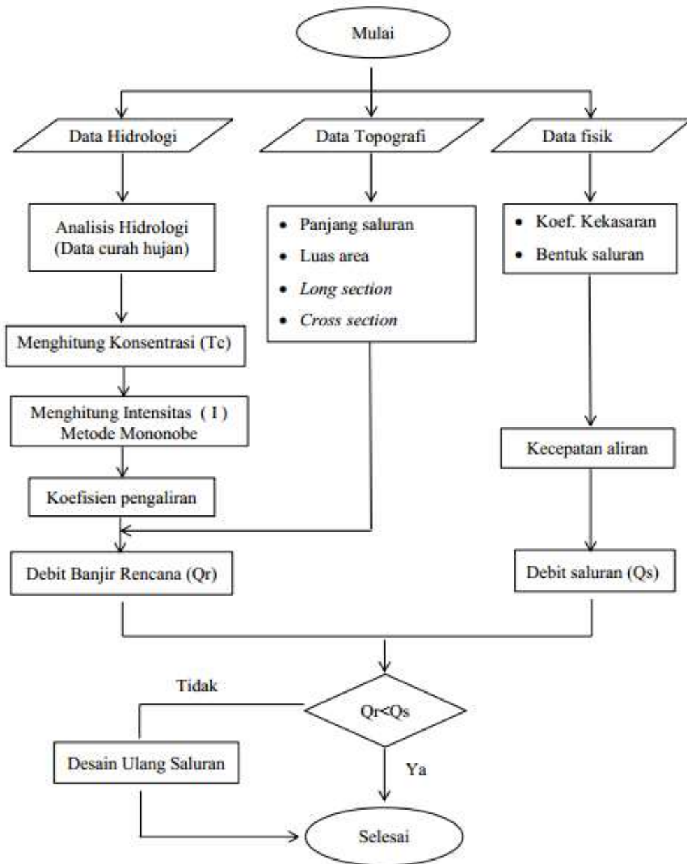
Gambar 3.4. Perencanaan Dimensi Saluran Drainase
