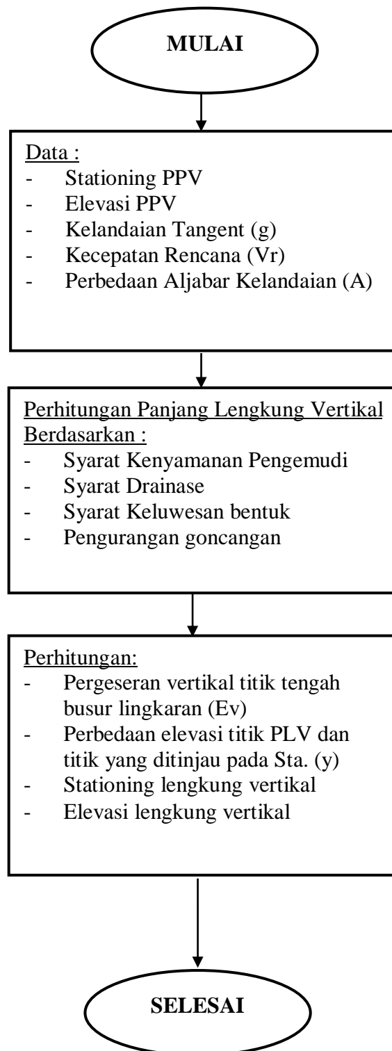
Gambar 3.2. Bagan Alir Perhitungan Alinemen Vertikal
