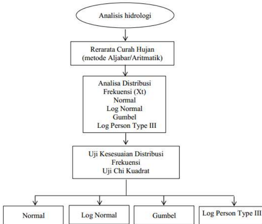
Gambar 3.3. Analisis Hidrologi
