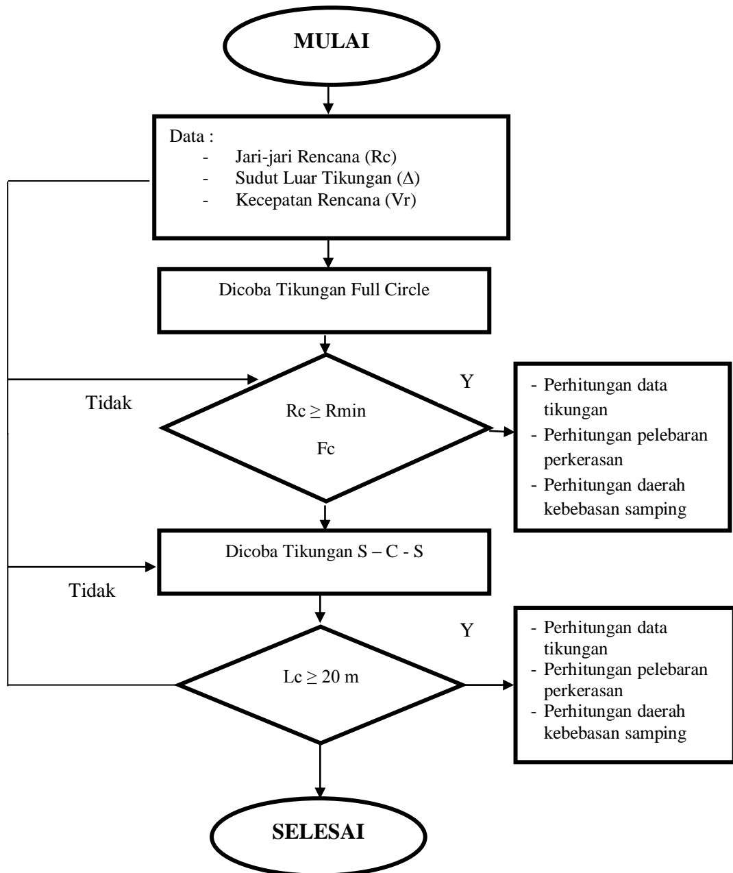
Gambar 3.1. Bagan Alir Perhitungan Alinemen Horizontal
