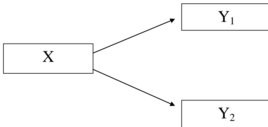
Gambar 3.2 Desain Penelitian
