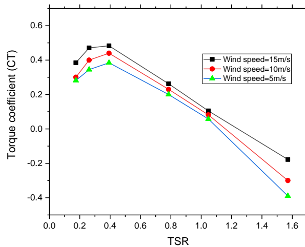
Fig. 20 Torque vs. TSR
