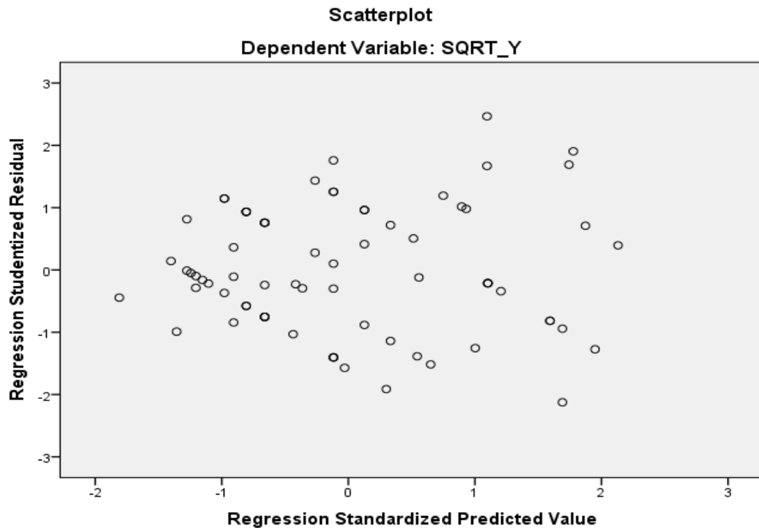
Gambar 4.1 Uji Heteroskedastisitas
