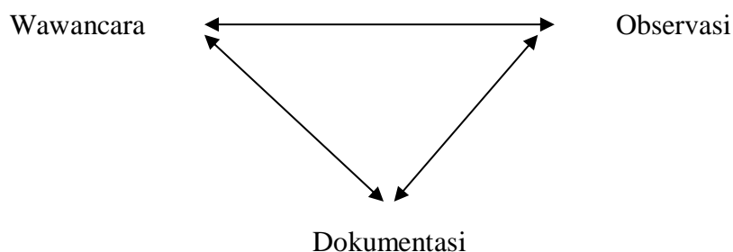
Gambar 3. 1 Triangulasi Sumber
