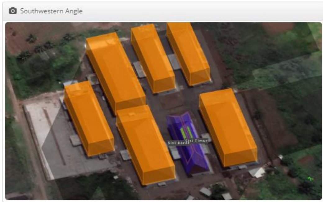
Pemodelan PLTS 15,4 kWp Array Kedua Sisi Atap
