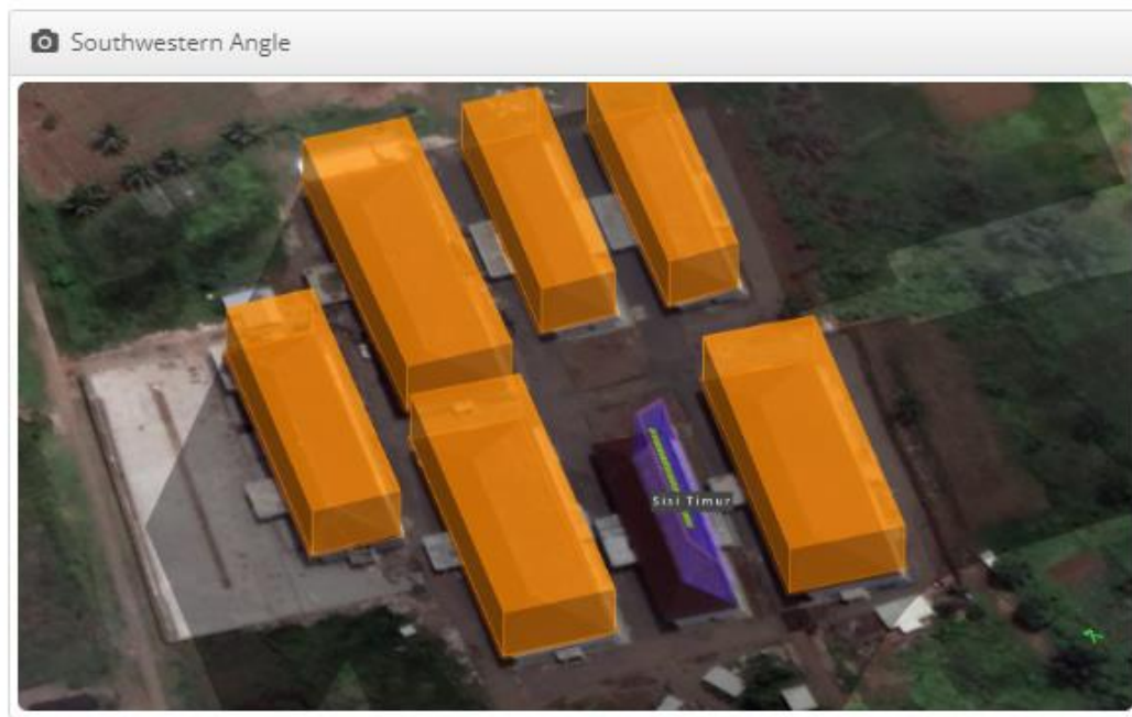
Pemodelan PLTS 15,4 kWp Array Atap Timur
