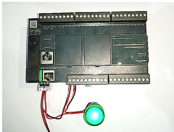
Gambar 2 Dokumentasi Pengujian Output PLC
