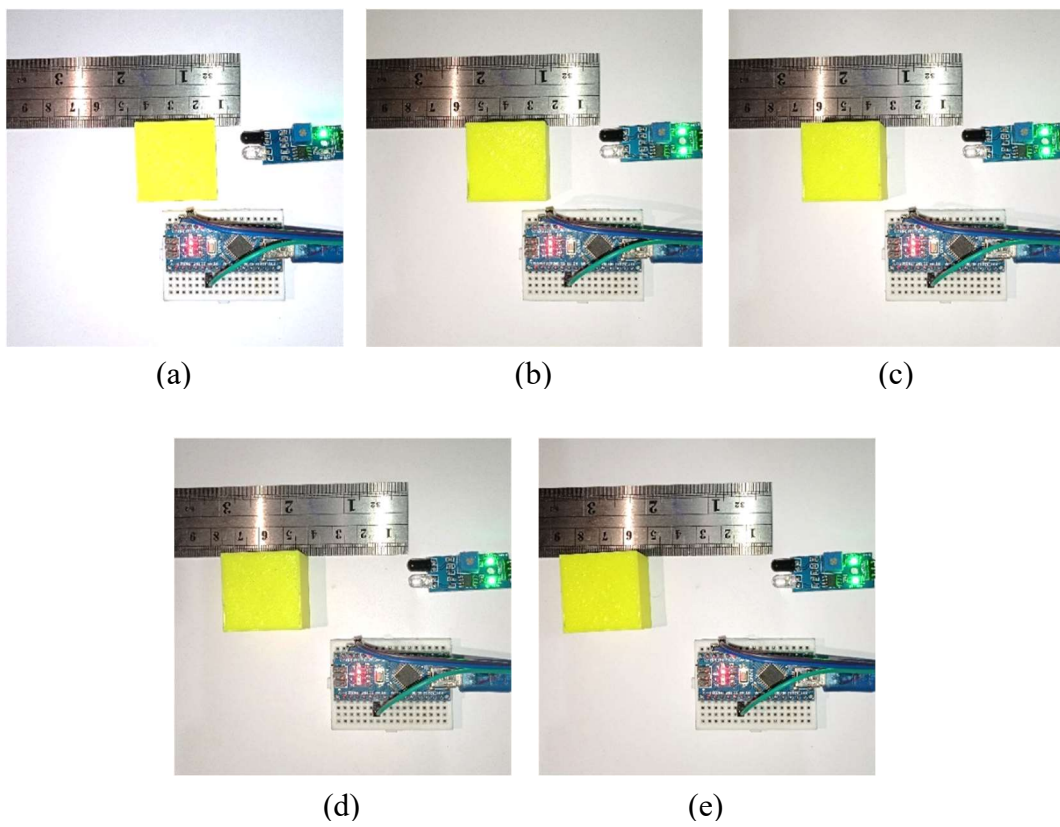
Gambar 9 Dokumentasi Pengujian Unit Photoelectric Sensor
