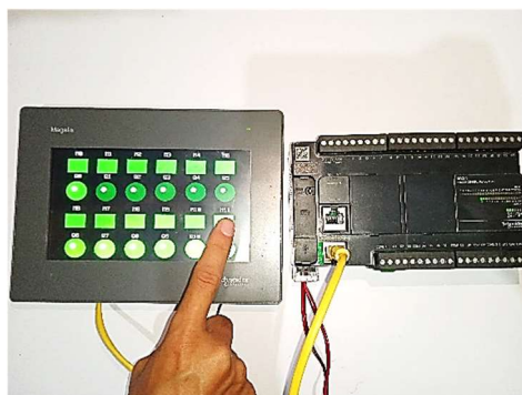
Gambar 5 Dokumentasi Pengujian Unit HMI
