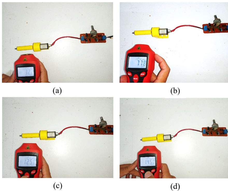
Gambar 7 Dokumentasi Pengujian Unit Motor DC dengan Mengukur Kecepatan pada tegangan; (a) 3 VDC, (b) 6 VDC, (c) 9 VDC, dan (d) 12 VDC
