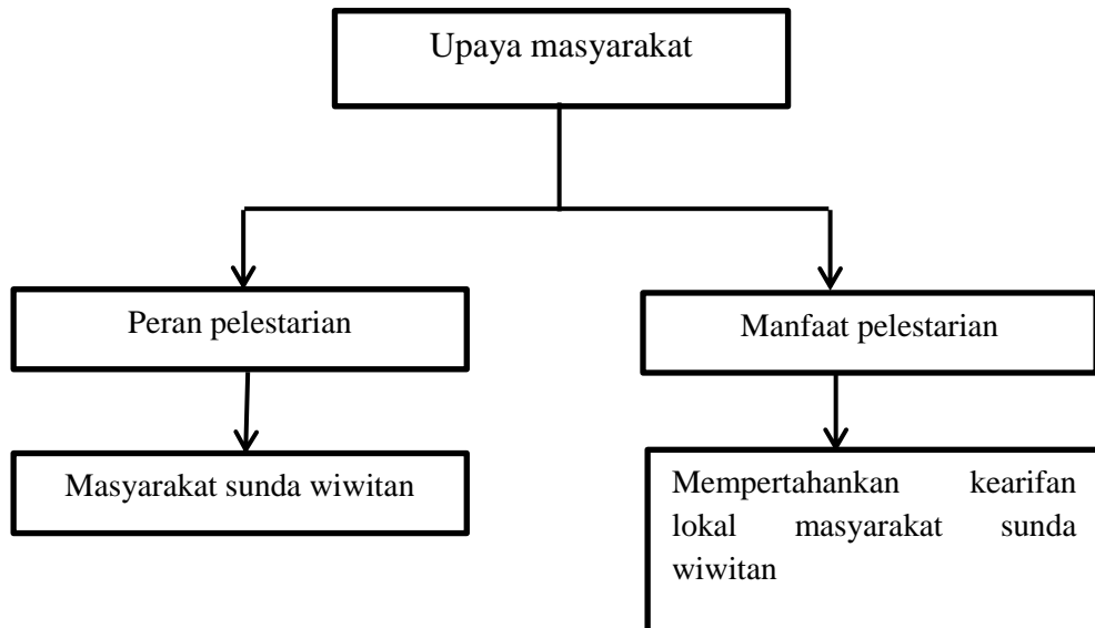
Gambar 2.2 Kerangka Konseptual 2
