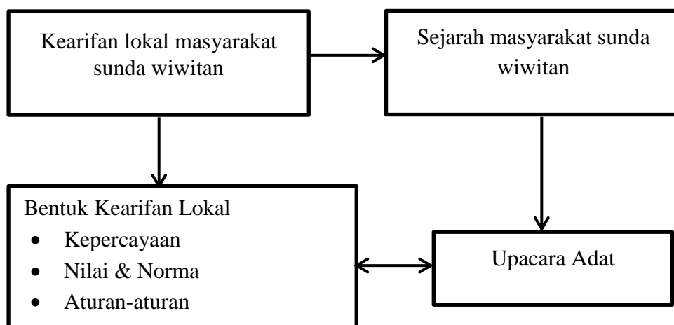
Gambar 2.1 Kerangka Konseptual 1
