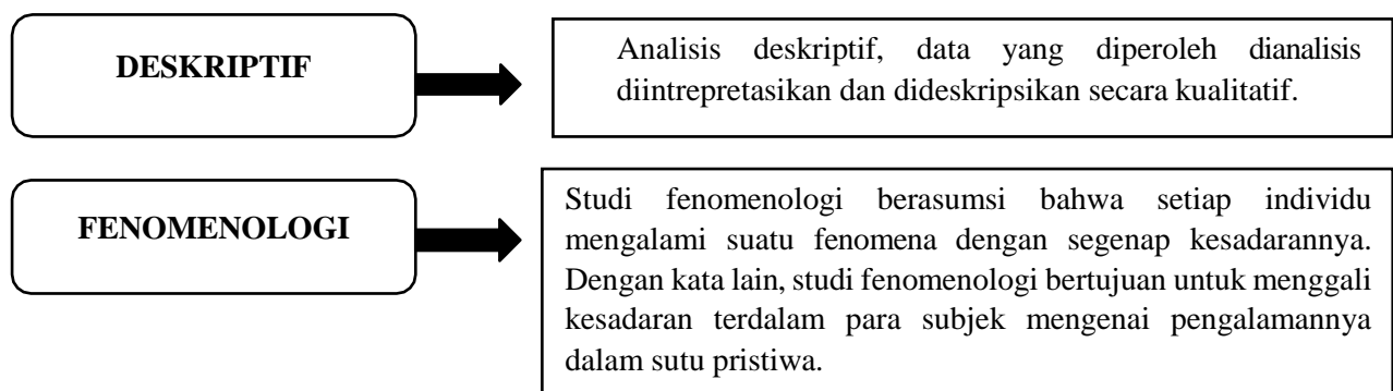
Gambar 3.1 Diagram Teknik Analisis Data
