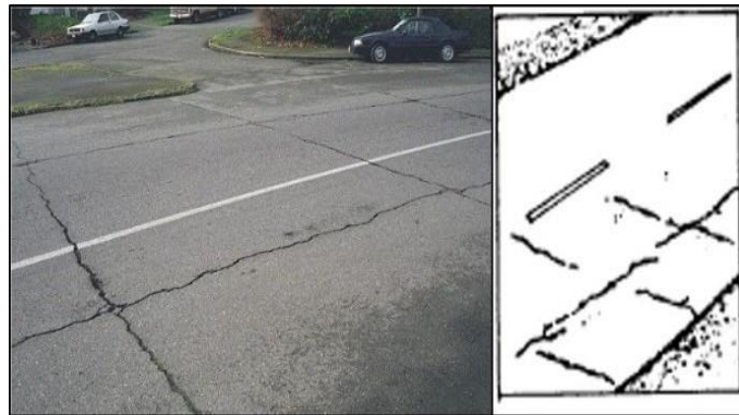
Gambar 2.13 Retak Kotak-kotak ( Block Cracking )
