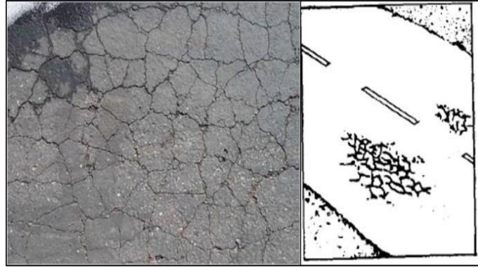
Gambar 2.9 Retak Kulit Buaya ( Alligator Cracking )
