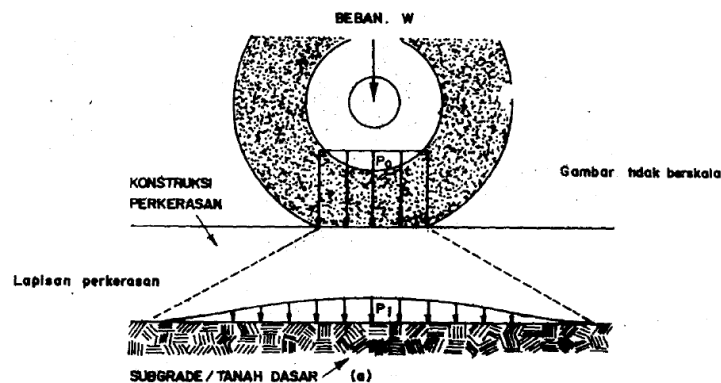
Gambar 2.8 Penyebaran Beban Roda Melalui Lapisan Perkerasan Jalan
