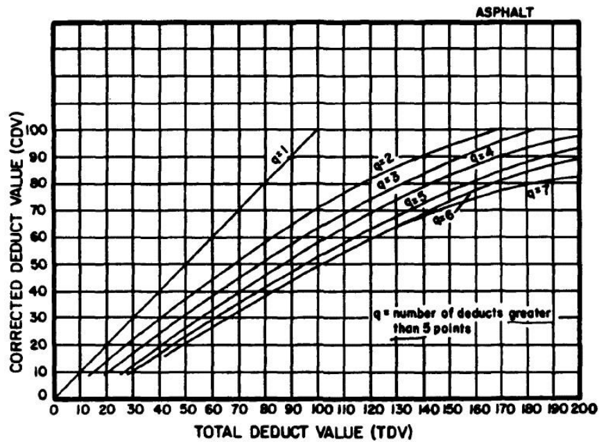
Gambar 2.41 Koreksi Kurva untuk Jalan dengan Perkerasan Aspal
